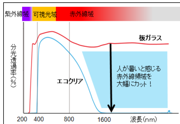
(表1 分光透過率)
